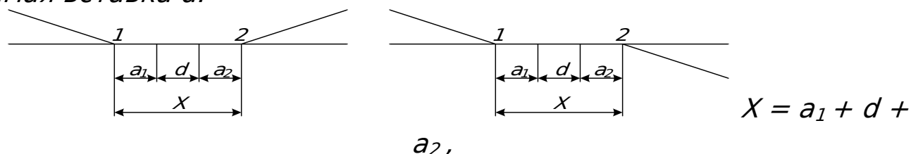
Рисунок 4 Схемы взаимного расположения стрелочных переводов при встречной укладке.
