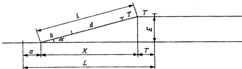
Рисунок 1 Конечное соединение:
