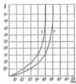
Рис. 22. Условия устойчивого горения дуги переменного тока для цепи, имеющей индуктивное и активное сопротивления (по С. Н. Тельяку и И. Т. Жарикову): 1 — равномерная дуга; 2 — прерывистая дуга.
