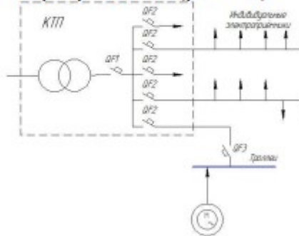
Рис. 1.3 Радиальная схема питания электроприемников
