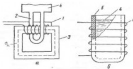
Рис. 23. Принципиальные схемы индукционного нагрева: а — схема печи с железным сердечником; б — схема печи без сердечника; 1 — первичная обмотка (индуктор); 2 — катушка, выходящий металл; 3 — железный сердечник; 4 — металлический инвентарь; 5 — футеровка печи (тегел)
