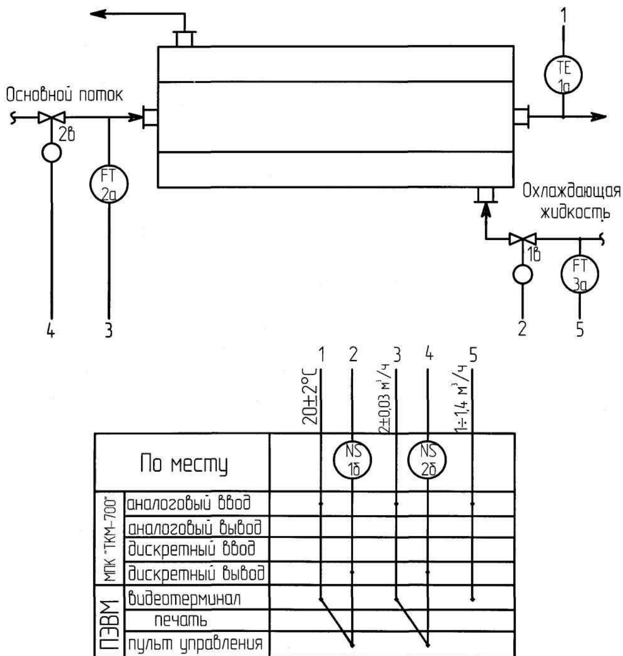
Рис. 14. Развернутая схема автоматизации теплообменника
