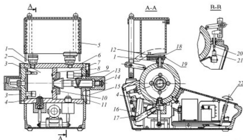
Рис. 13.3. Устройство стенда ОТ 17 для определения величины тушающего зазора:
