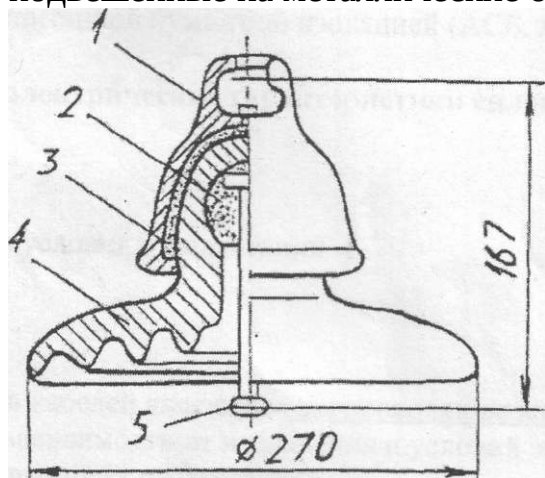
Рис. 5 Подвесной изолятор
