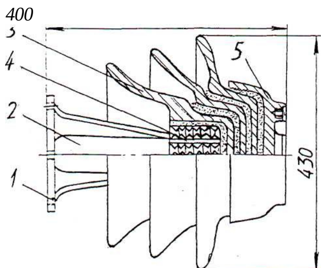
Рис 2. Опорно - штыревой изолятор.
