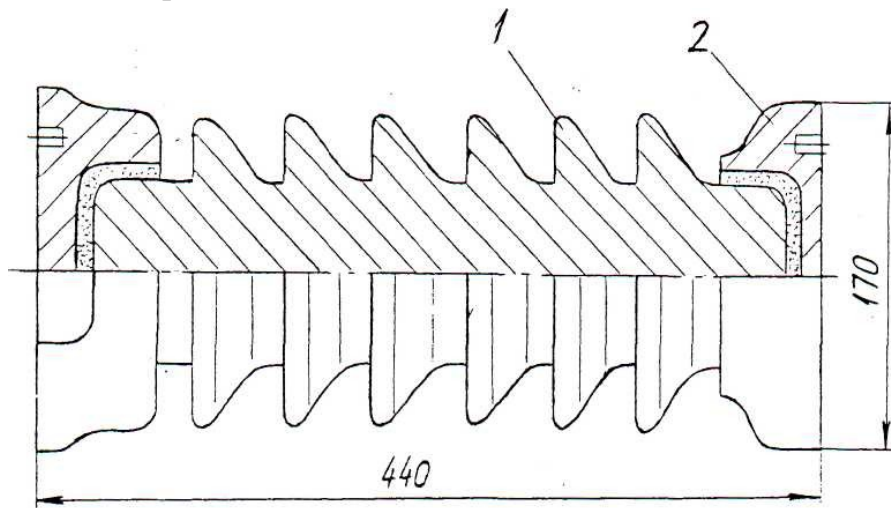
Рис. 3 Опорно - стержневой изолятор.
