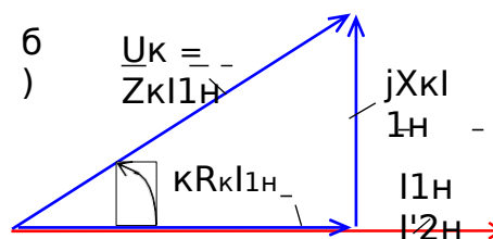
Рис.6. Схема первичной обмотки трансформатора и векторная диаграмма напряжений на ней в режиме КЗ.
