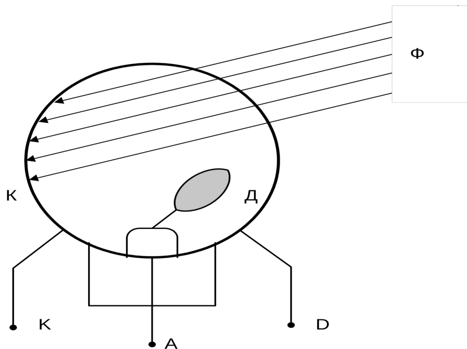
Рис.1.6. Схема фотоэлемента с усилением фототока. К - катод; Д - динод; А - анод, Ф - световой поток
