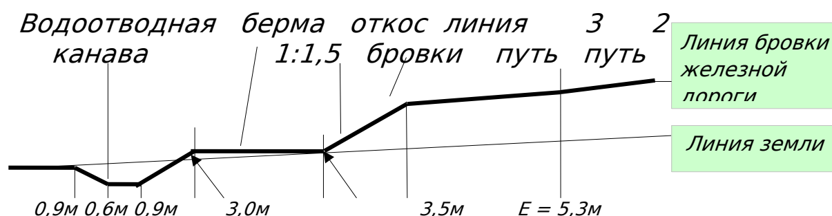
Рисунок 6 Часть поперечного профиля
