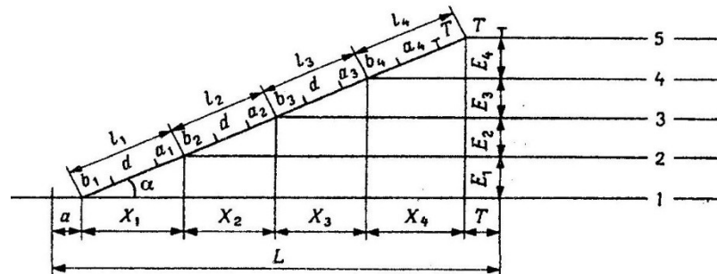
Рисунок 3 Стрелочные улицы под углом крестовины.
