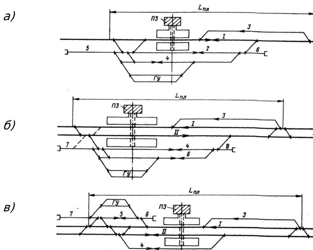
Рисунок 10 Схемы промежуточных станций с полупродольным расположением путей:
