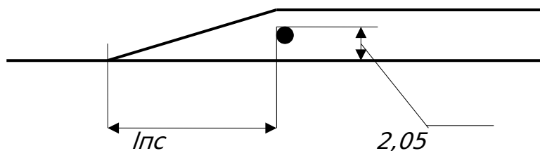
Рисунок 1 Схема установки предельного столбика в междупутье
