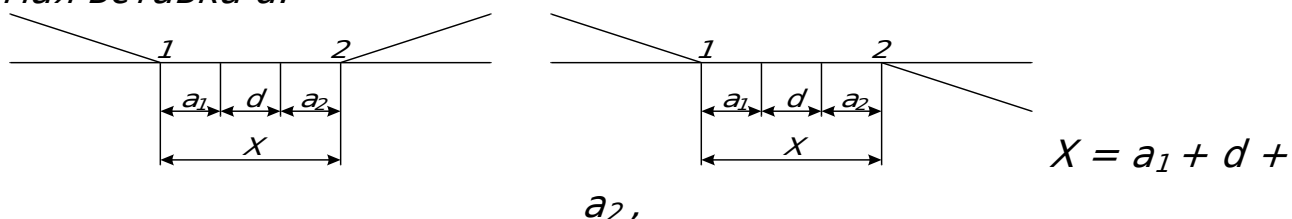
Рисунок 4 Схемы взаимного расположения стрелочных переводов при встречной укладке.
