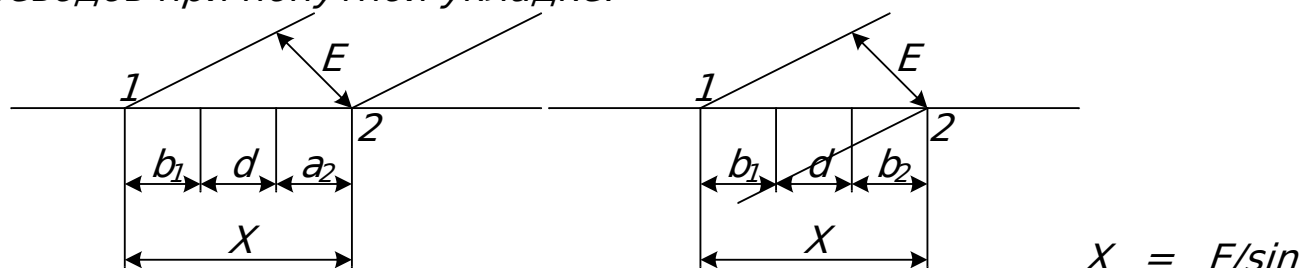
Рисунок 5 Схемы взаимного расположения стрелочных переводов при попутной укладке.
