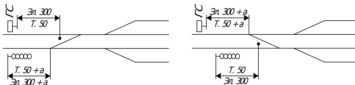
Рисунок 2 Установка входных светофоров: а- противошерстный стрелочный перевод, б- пошерстный стрелочный перевод.
