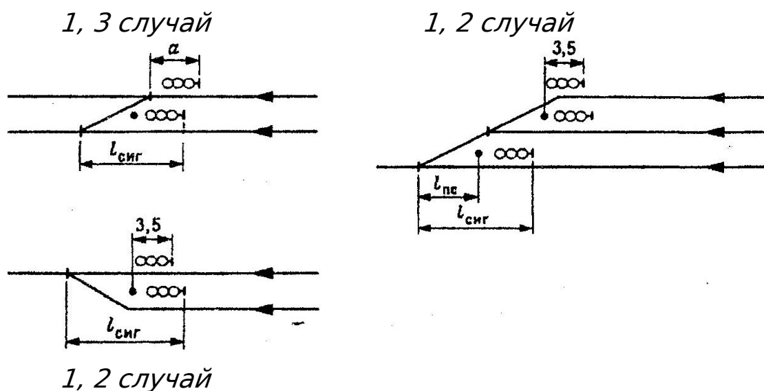
Рисунок 3 Установка выходных светофоров
