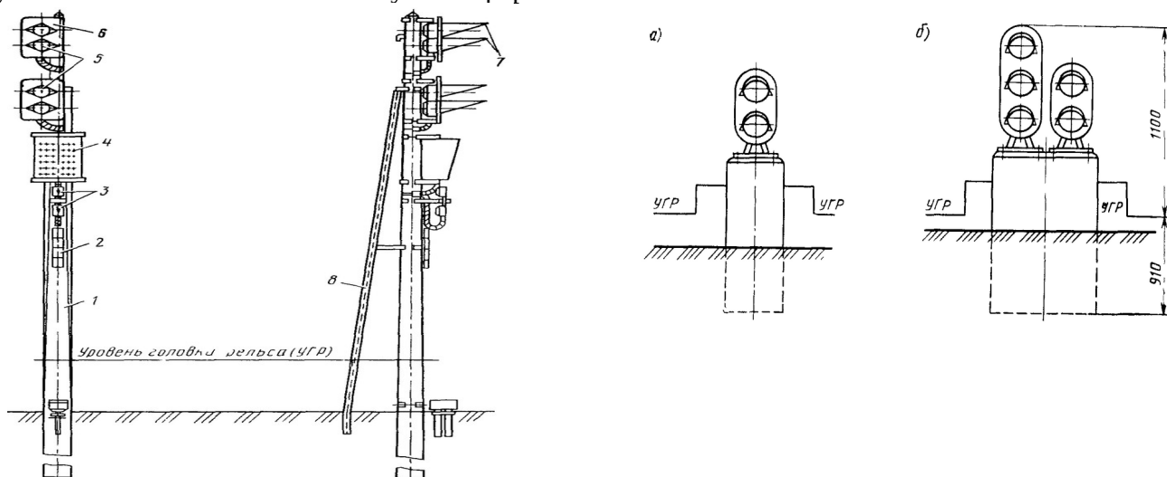
Рисунок 3.1 - Железнодорожные светофоры.
