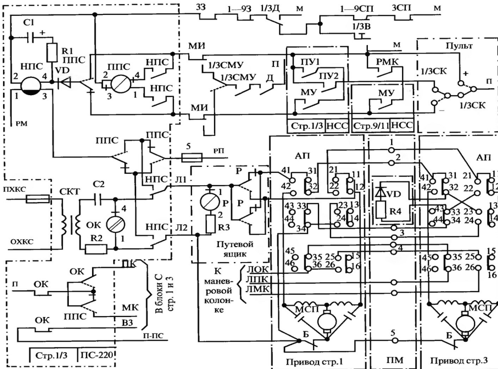
Рисунок 1 - Двухпроводная схема управления спаренной стрелкой
