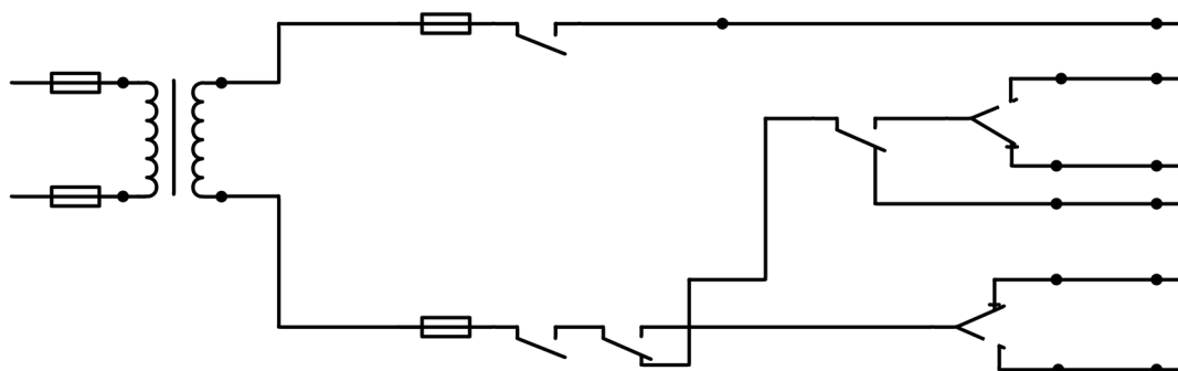
Рисунок 3.1 - Принципиальная схема
