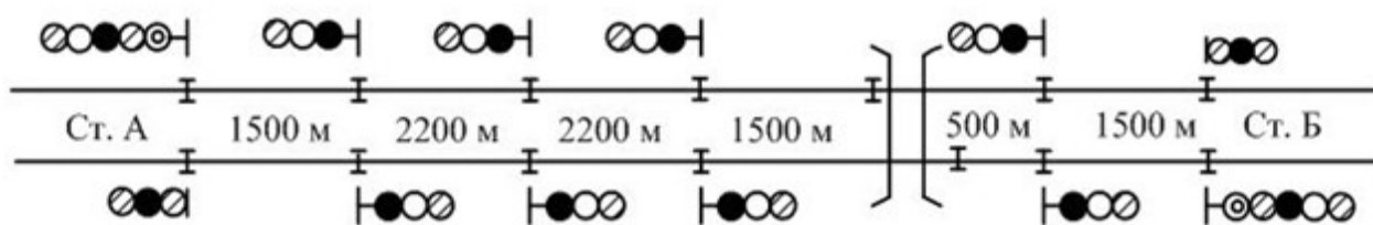
Рисунок 1 - Путевой план перегона
