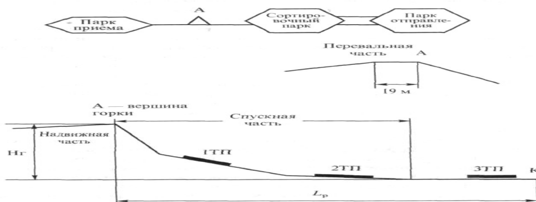
Рисунок 2 - Схема сортировочной горки
