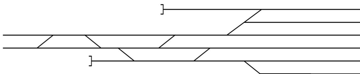
Рисунок 1- Схема горловины станции
