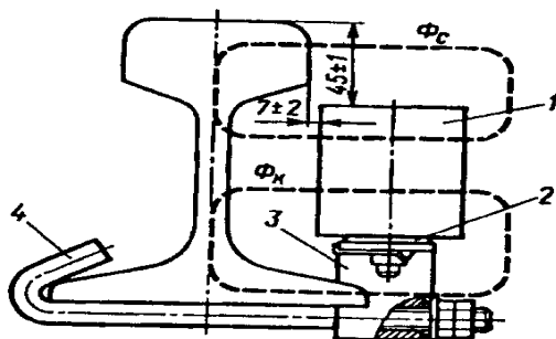
Рисунок 2.1 - Путевой датчик ДП50-80
