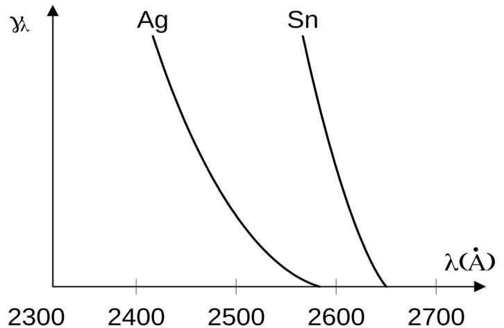
Рис.1.4. Спектральная чувствительность y_\lambda фотокатода
