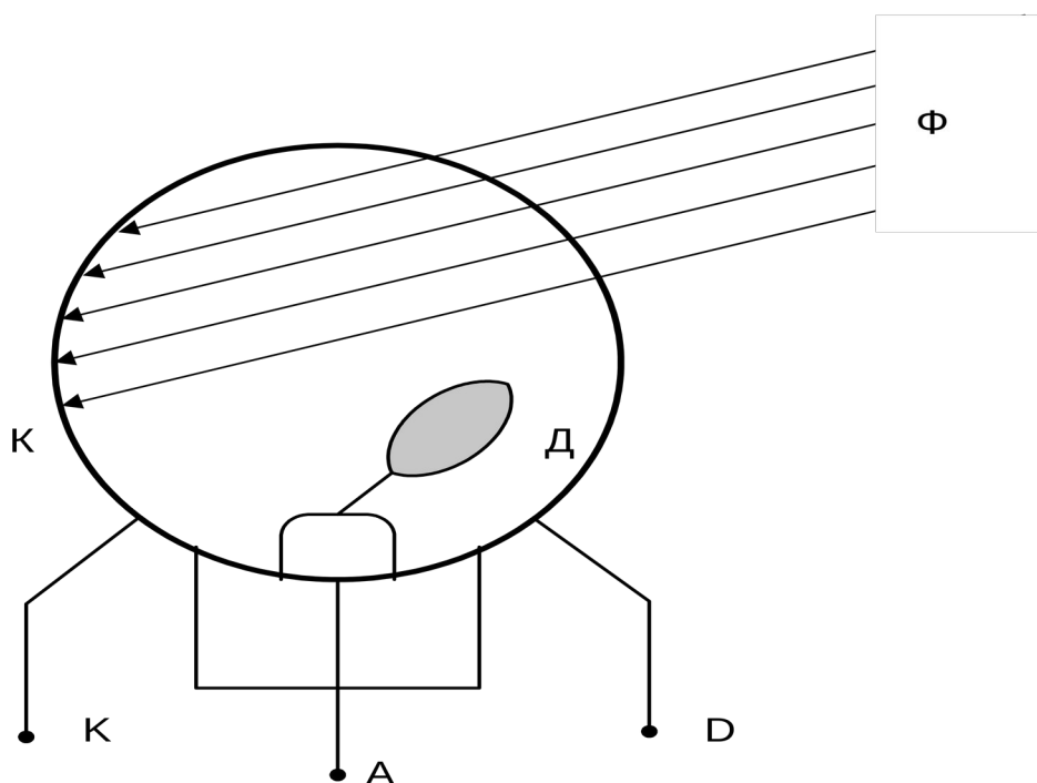
Рис.1.6. Схема фотоэлемента с усилением фототока.
