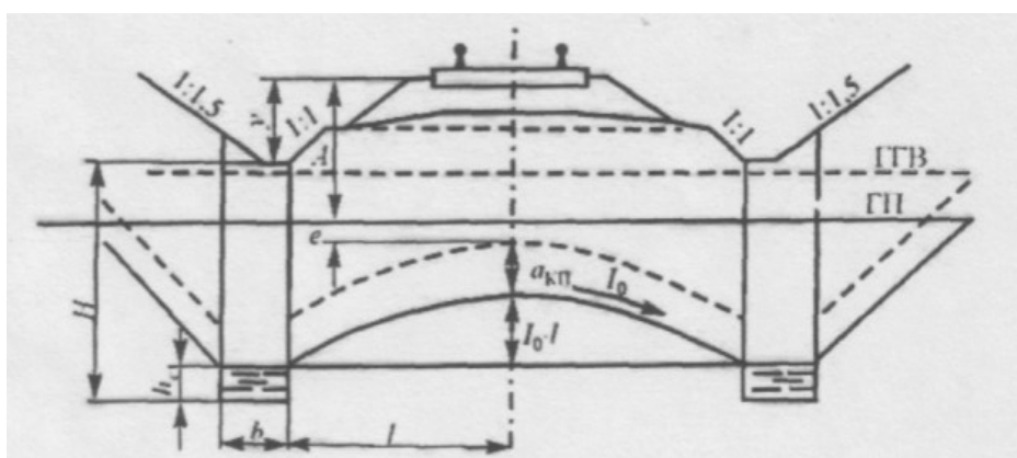
Рис.3.2 Схема двустороннего подкюветного дренажа, «ГТВ» - уровень грунтовых вод до устройства дренажа,
