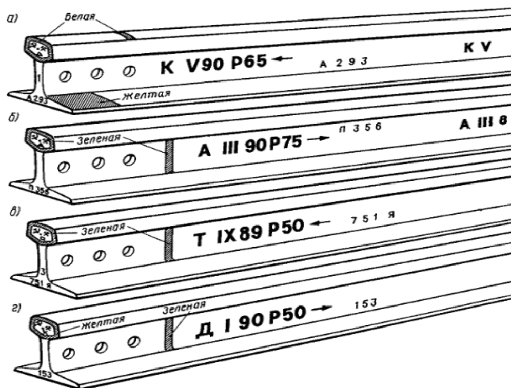
Рис. 4.1 Маркировка рельсов
