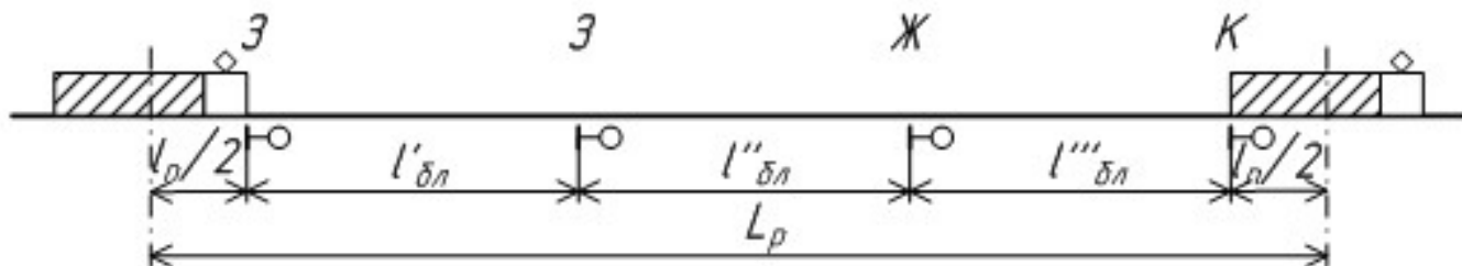
Рисунок 1 Разграничение поездов тремя блок-участками
