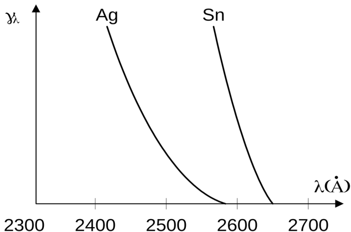
Рис.1.4. Спектральная чувствительность y\lambda фотокатода
