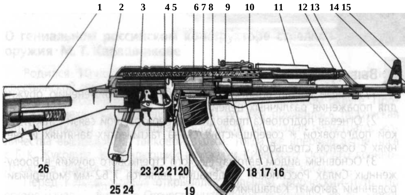
Рис. 1. 7,62-мм АКМ:
