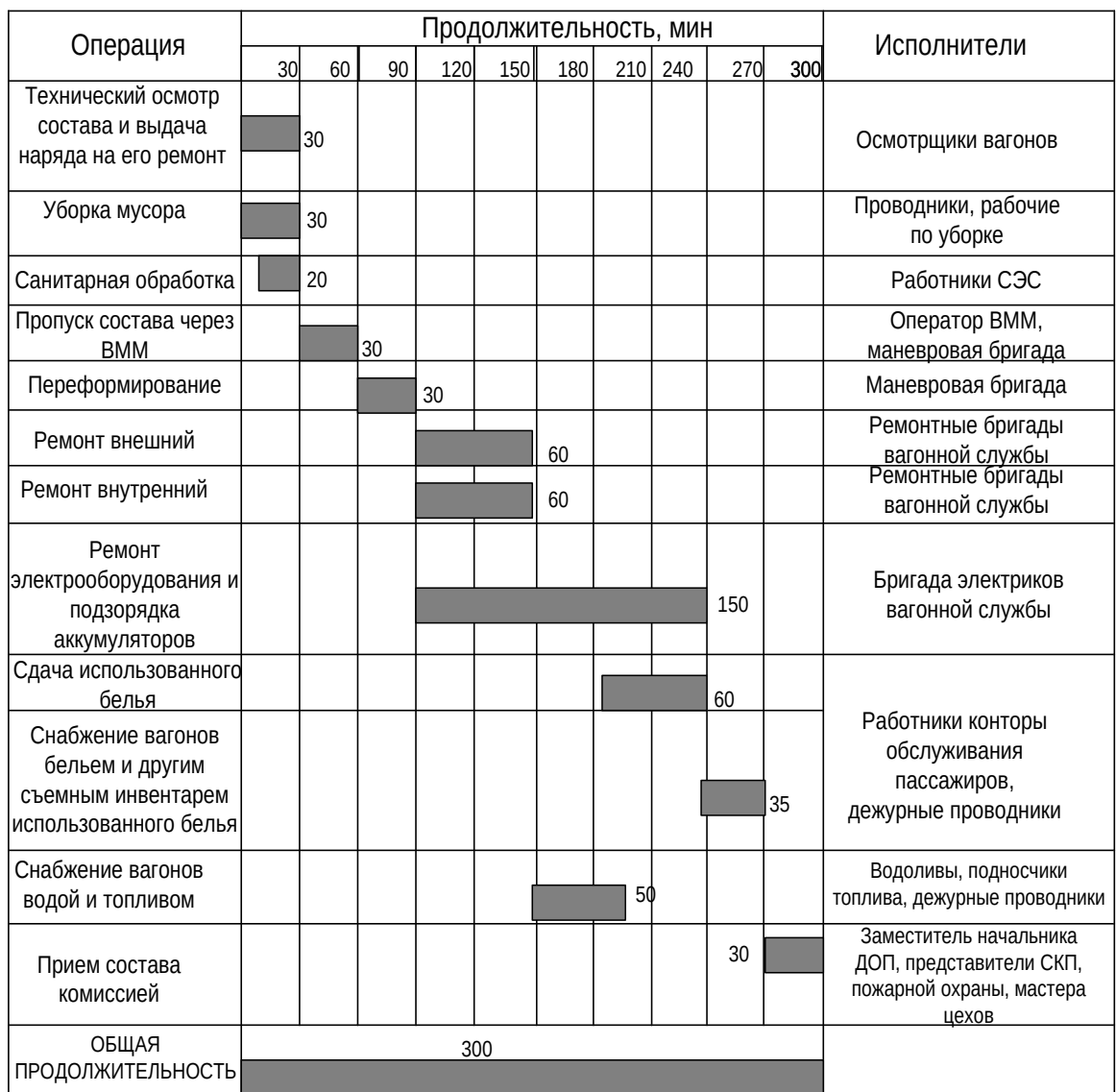
Рис. 1. График операций по обработке состава фирменного скорого поезда в пункте формирования
