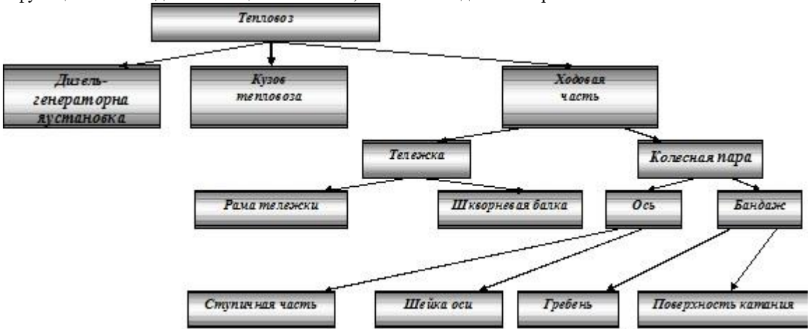
Рис 1 Блочно—функциональная декомпозиция Этап 2 Выбор методов диагностирования
