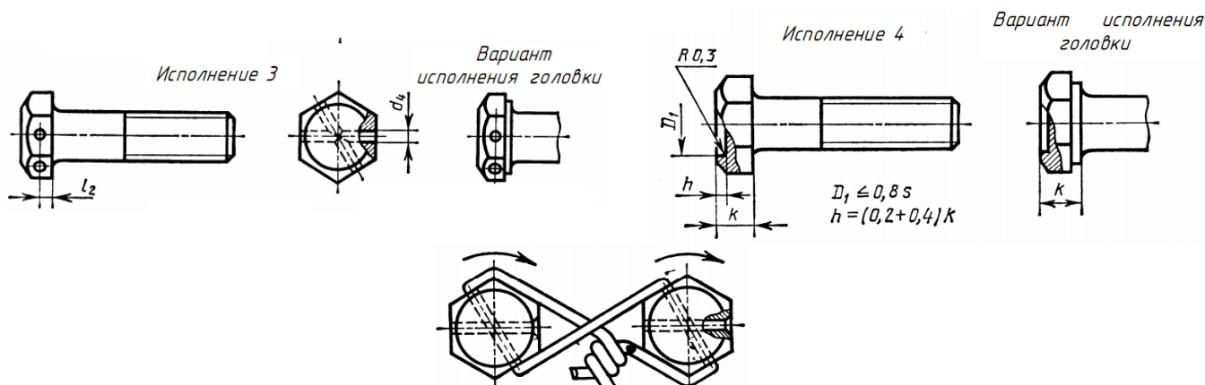
Рисунок 8 Исполнения болтов с шестигранной головкой
