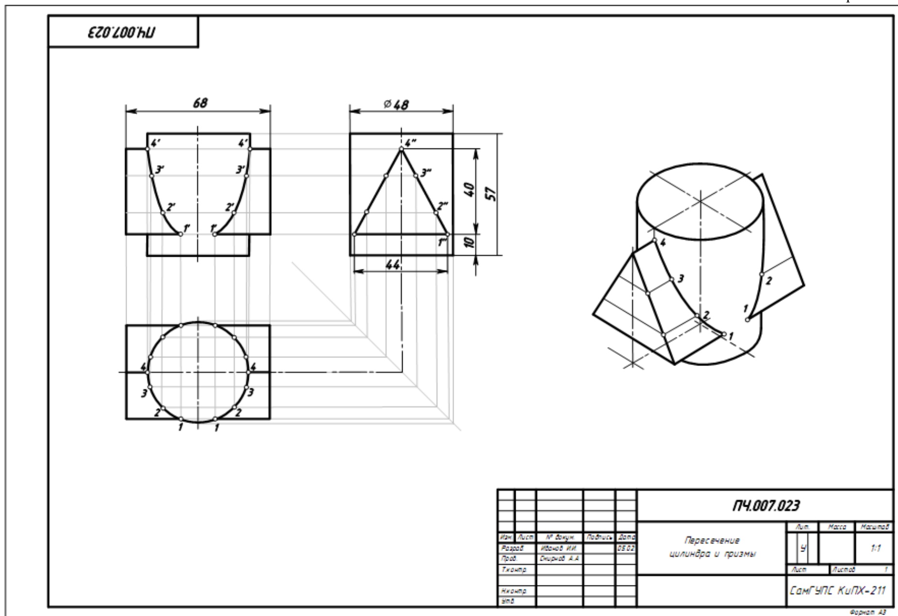
Рисунок 5.1 Образец выполнения чертежа «Пересечение цилиндра и призмы»
