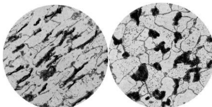
Рисунок 1– Микроструктуры стали после холодной деформации и после рекристаллизации
