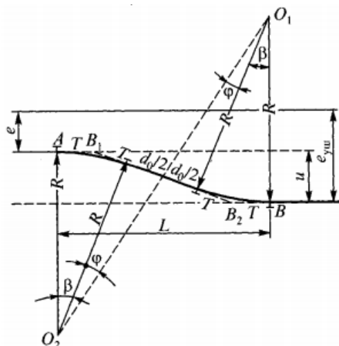
Рисунок 6.1 – Схема раздвижки путей с параллельным смещением одного из них при изменении величины междупутья
