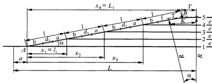
Рисунок 4.1 –Схема простейшей стрелочной улицы под углом крестовины
