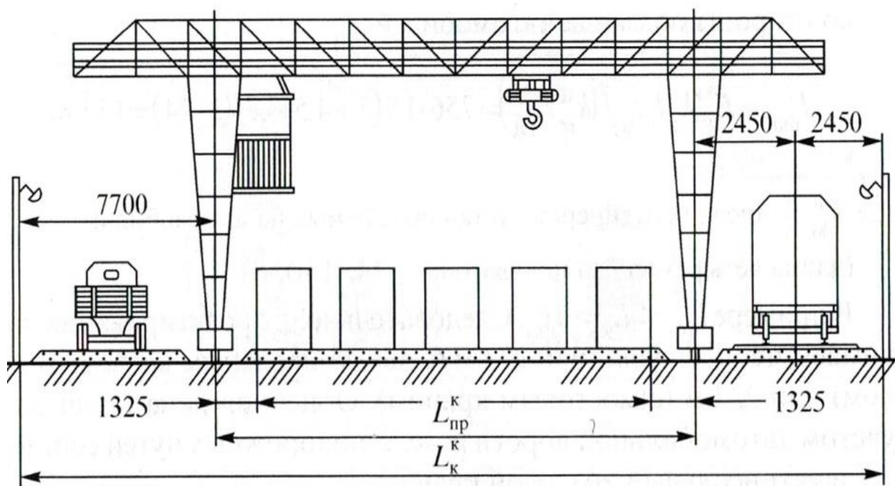
Рисунок 11.1 - Схема механизации переработки контейнеров
