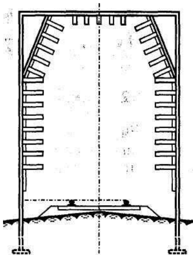
Рисунок 6 – Габаритные ворота
