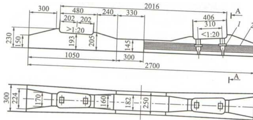
Рис. 9. Железобетонная шпала типа Ш1
