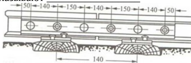
Рис. 2. Боковой вид стыка
