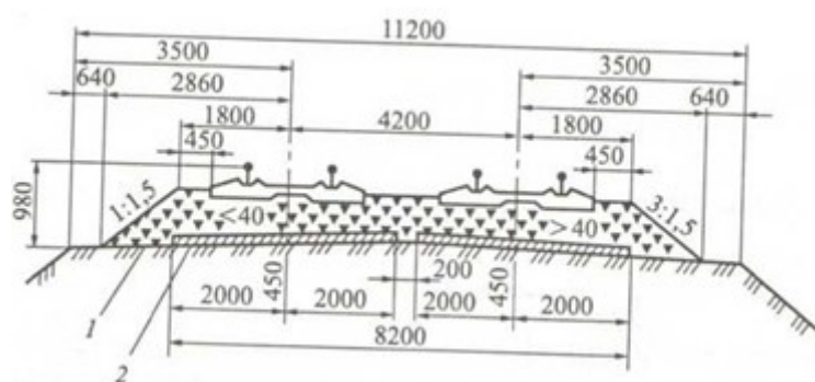
Рис. 10. Типовой поперечный профиль балластной призмы
