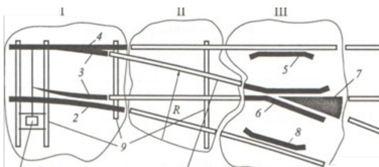
Рис.1. Обыкновенный стрелочный перевод
