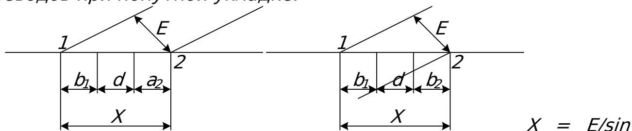
Рисунок 5 Схемы взаимного расположения стрелочных переводов при попутной укладке.
