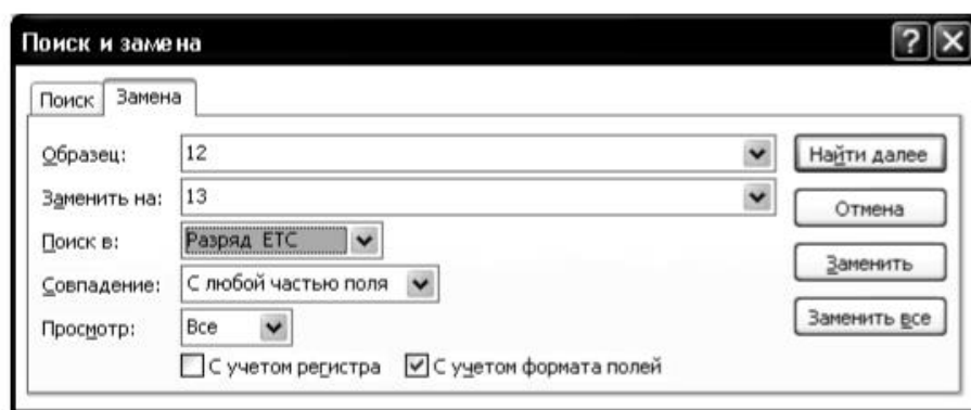
Рис. 11. Окно Замена
