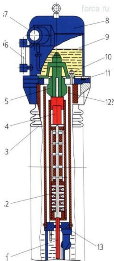
Рисунок 1 Основные элементы выключателя ВМТ-110 полюса.
