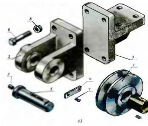
Рисунок 2 Составные части «Блока направляющего»
