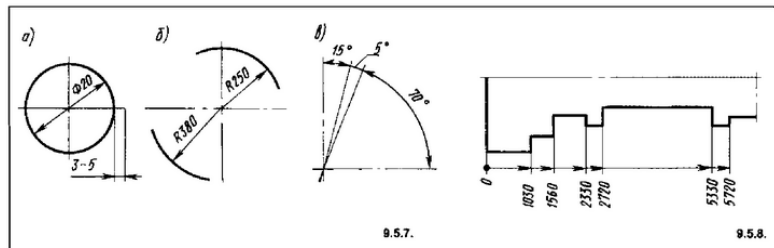
Рисунок 3 Нанесение отметок
