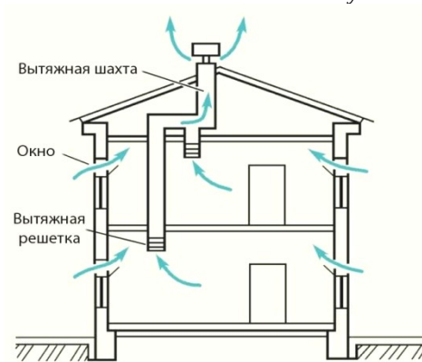
Схема естественной вентиляции Рисунок 2.1
