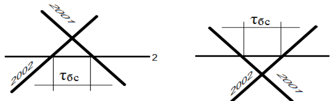
Рисунок 1 Расположение встречных поездов на двухпутной вставке при безостановочном их скрещении
