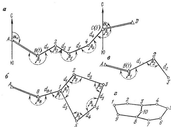
Рис. 56. Виды теодолитных ходов
