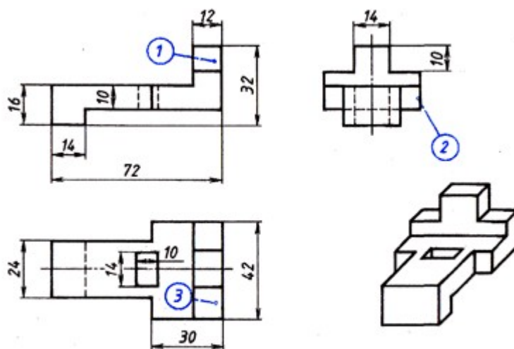
Рис. 148. Упор
