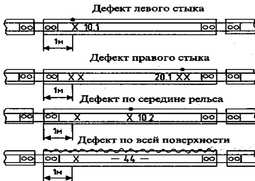
Рис 1 маркировка рельсов в пути (на перегоне)
