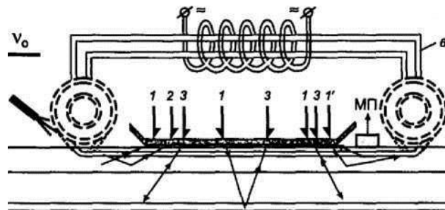
Рис 3.совмещенный вагон-дефектоскоп «АВИКОН-03»
