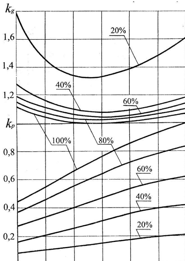
Рисунок 1 Безразмерная характеристика дизеля
