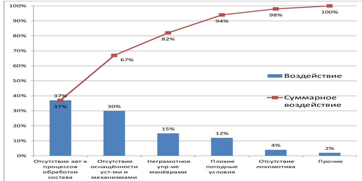
Рисунок 1 – Диаграмма Парето
